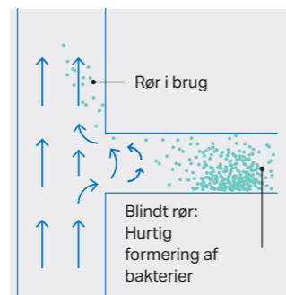
Blinde rør, hvor vandet ikke udskiftes, fremmer bakteriedannelsen.
