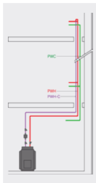
Konventionel cirkulation: separate rør til varmtvandsindløb og tilbageløb
