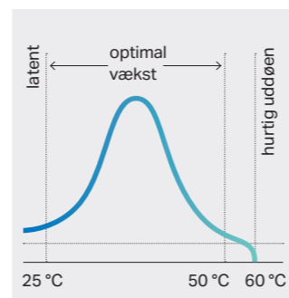
Legionella-bakterier reproduceres specielt hurtigt i vand ved temperaturer mellem 25 og 50 °C.
