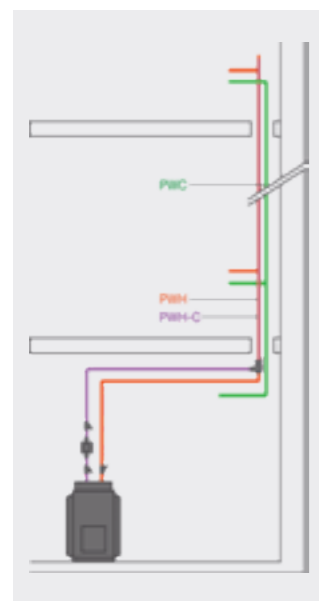
Indvendig cirkulation: sparer materiale, plads og energi.
